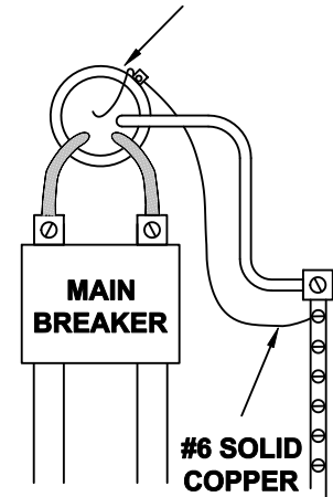
METAL CONDUIT GROUNDING BUSHING
