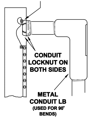
METAL CONDUIT GROUNDING BUSHING
